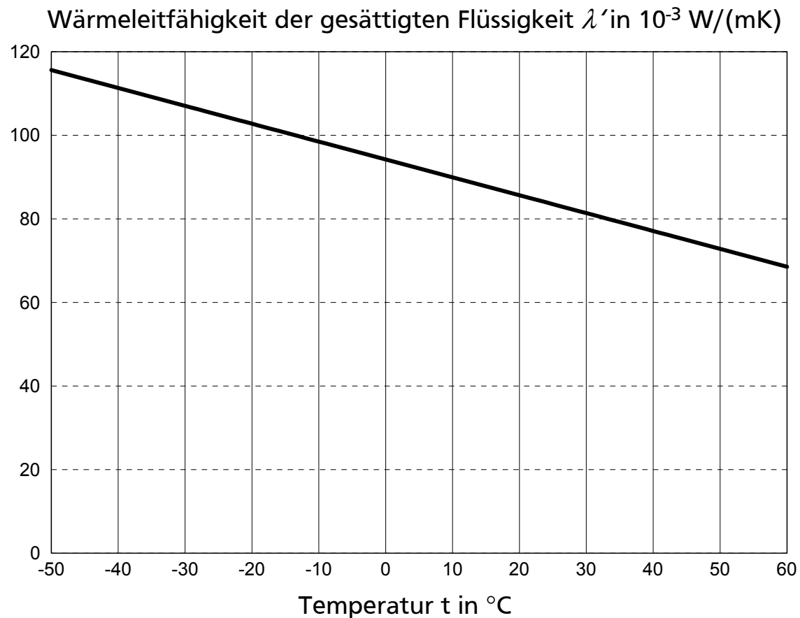
Abbildung 3: Wärmeleitfähigkeit der gesättigten Flüssigkeit
