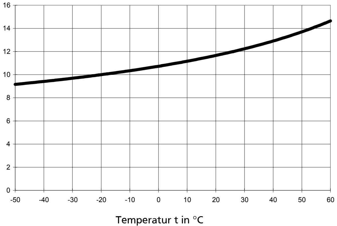
Abbildung 2: Dynamische Viskosität des gesättigten Dampfes
