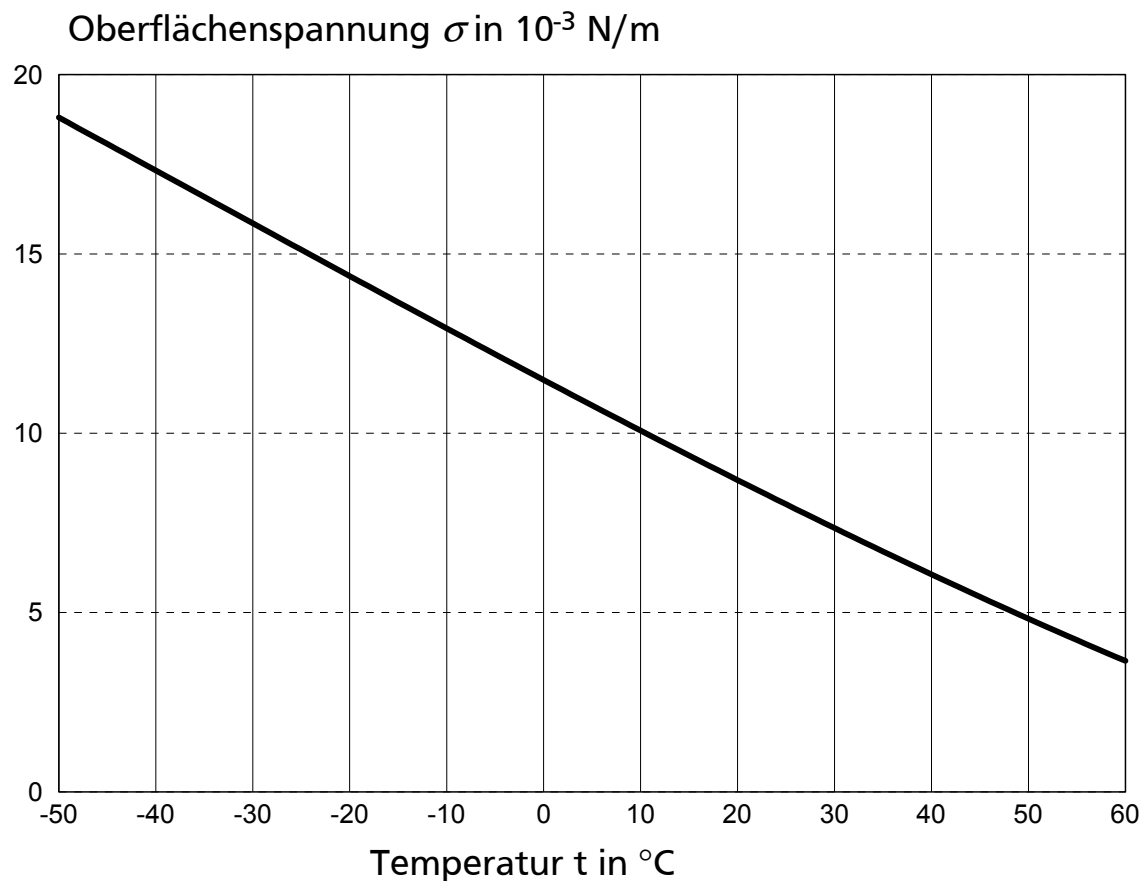
Abbildung 5: Oberflächenspannung
