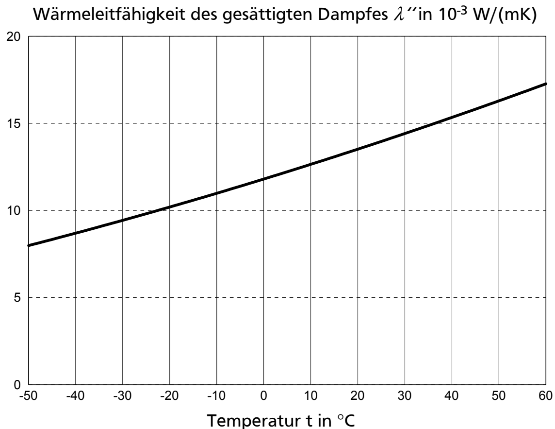
Abbildung 4: Wärmeleitfähigkeit des gesättigten Dampfes
