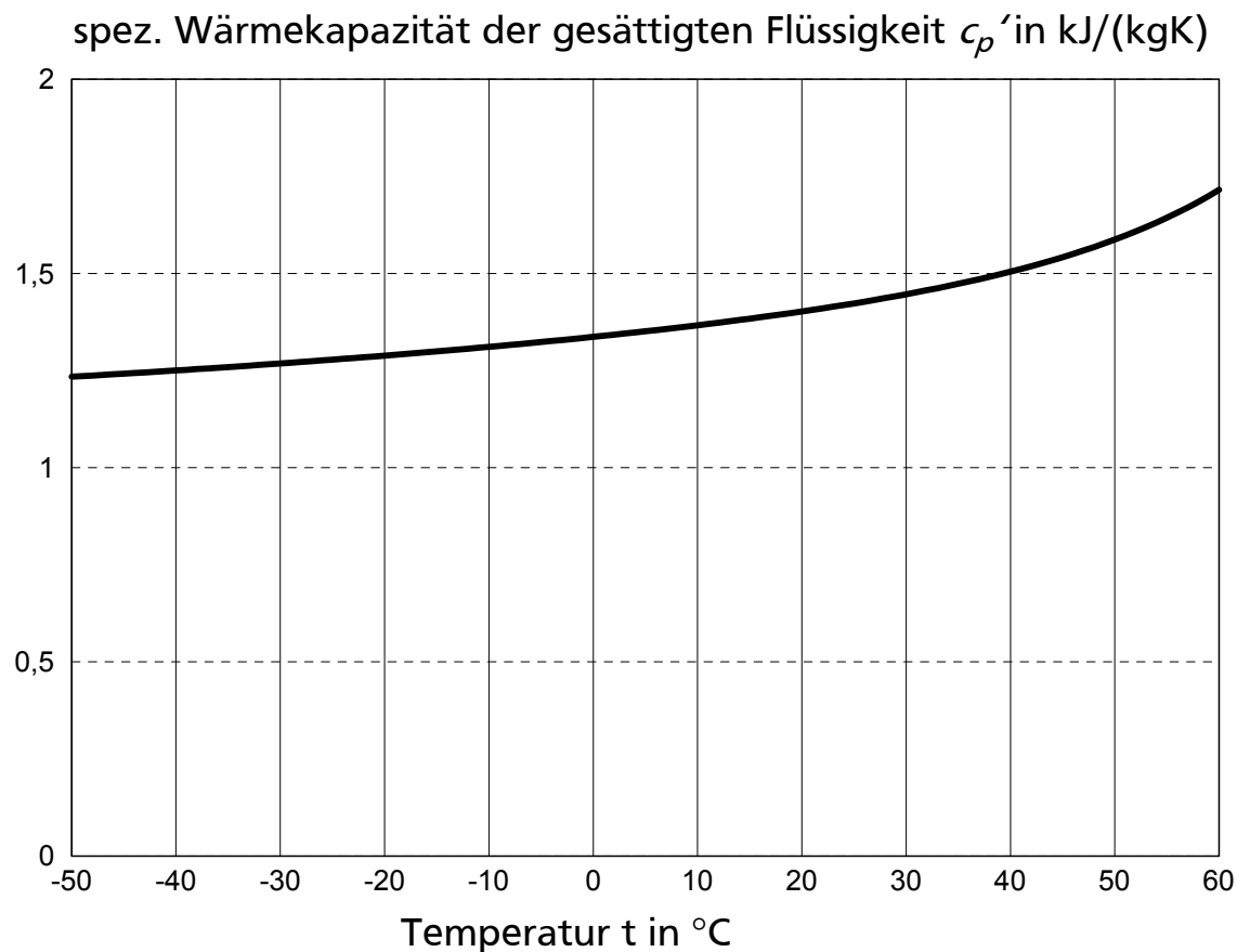
Abbildung 6: Spezifische Wärmekapazität der gesättigten Flüssigkeit
