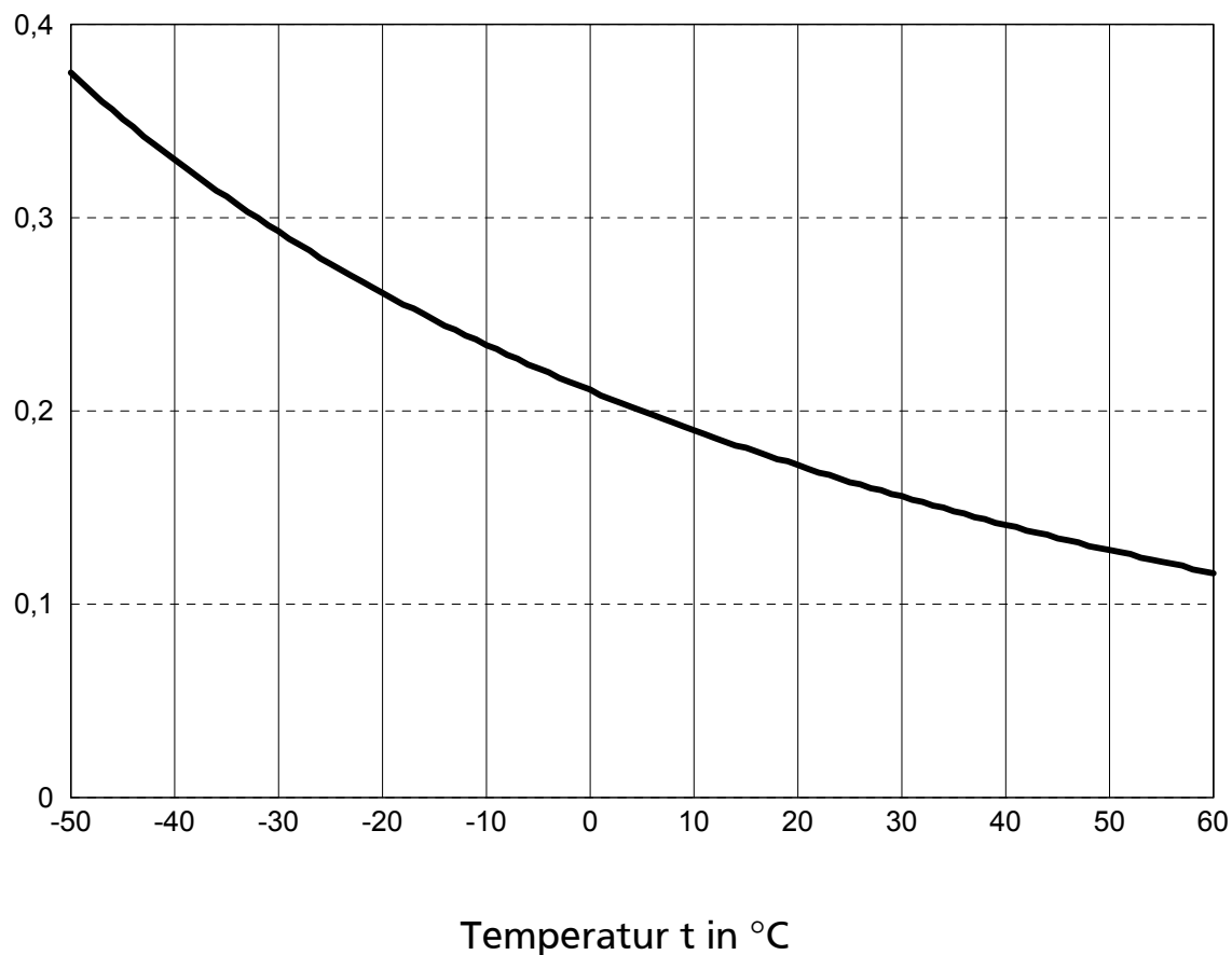
Abbildung 1: Dynamische Viskosität der gesättigten Flüssigkeit
